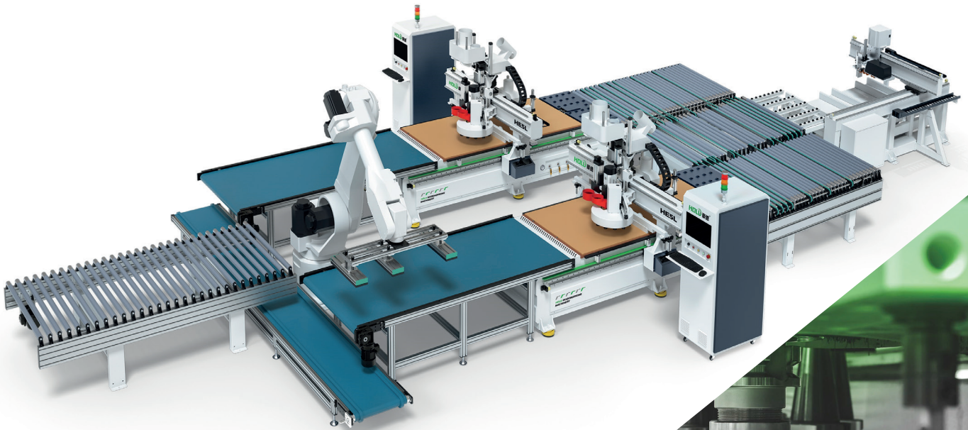
HOLD HE SERİSİ Düz tabla CNC işleme merkezi çözümleri / CNC working center - Nesting solutions
